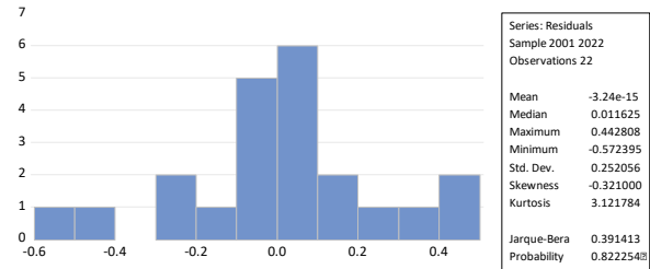
Gambar 4. Hasil Uji Normalitas
